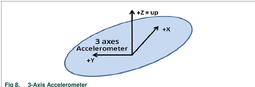
Fig 8. 3-Axis Accelerometer
