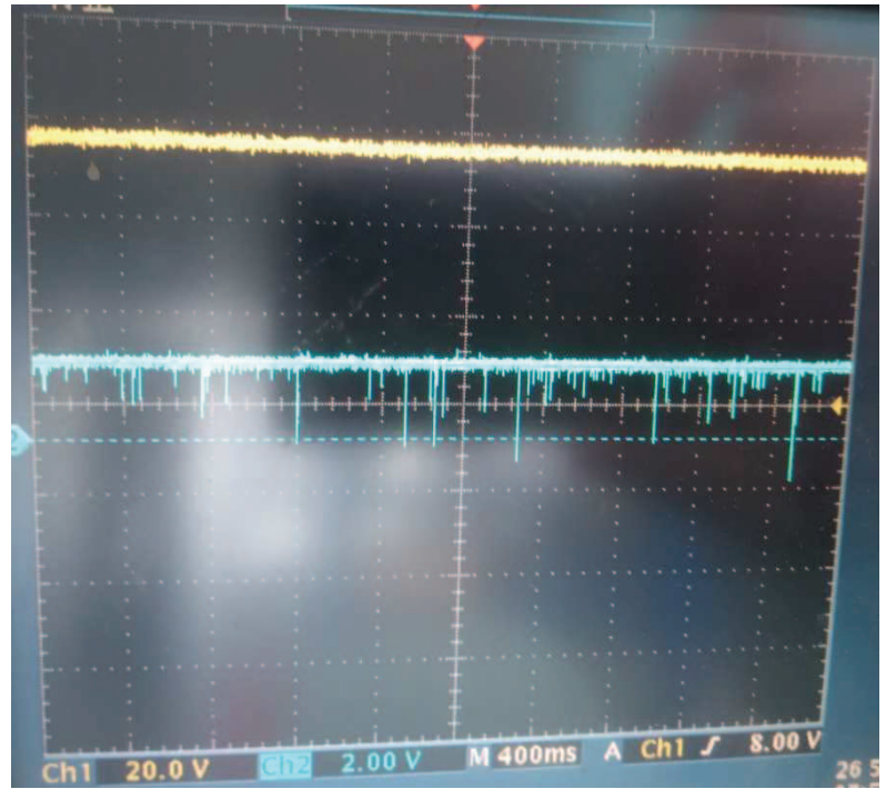
空载输出电压和TL431 REF波形
