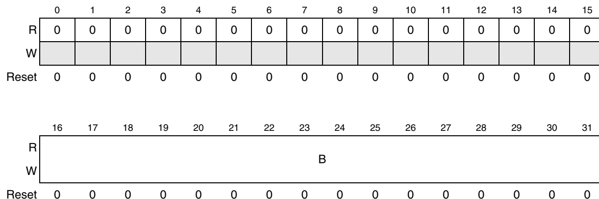
Figure 27-13. eMIOS UC B Register (EMIOSB[n])
