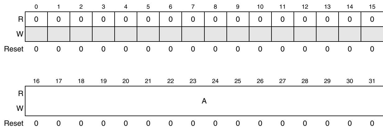
Figure 27-12. eMIOS UC A Register (EMIOSA[n])
