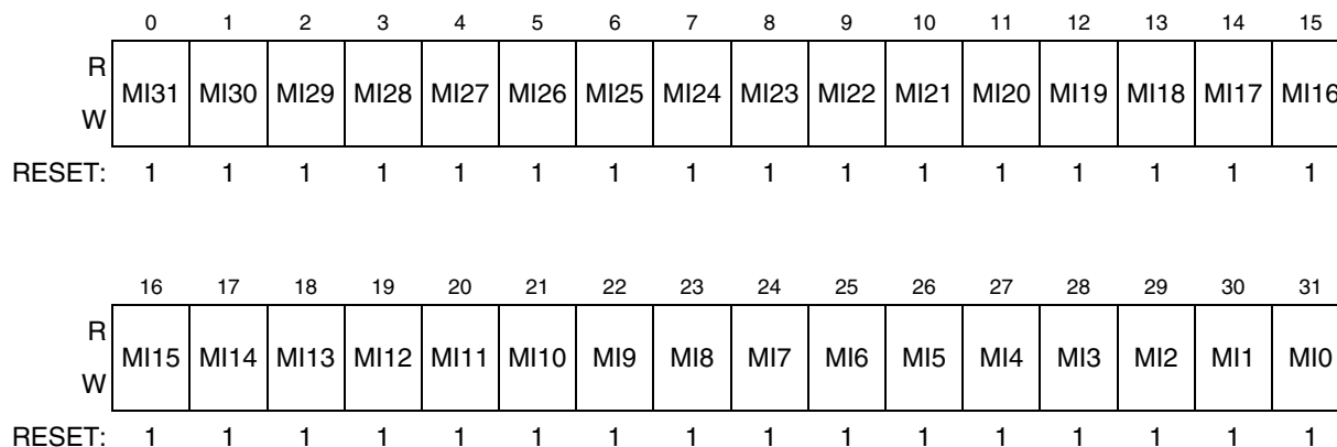
Figure 25-8. Rx Global Mask Register (RXGMASK)
