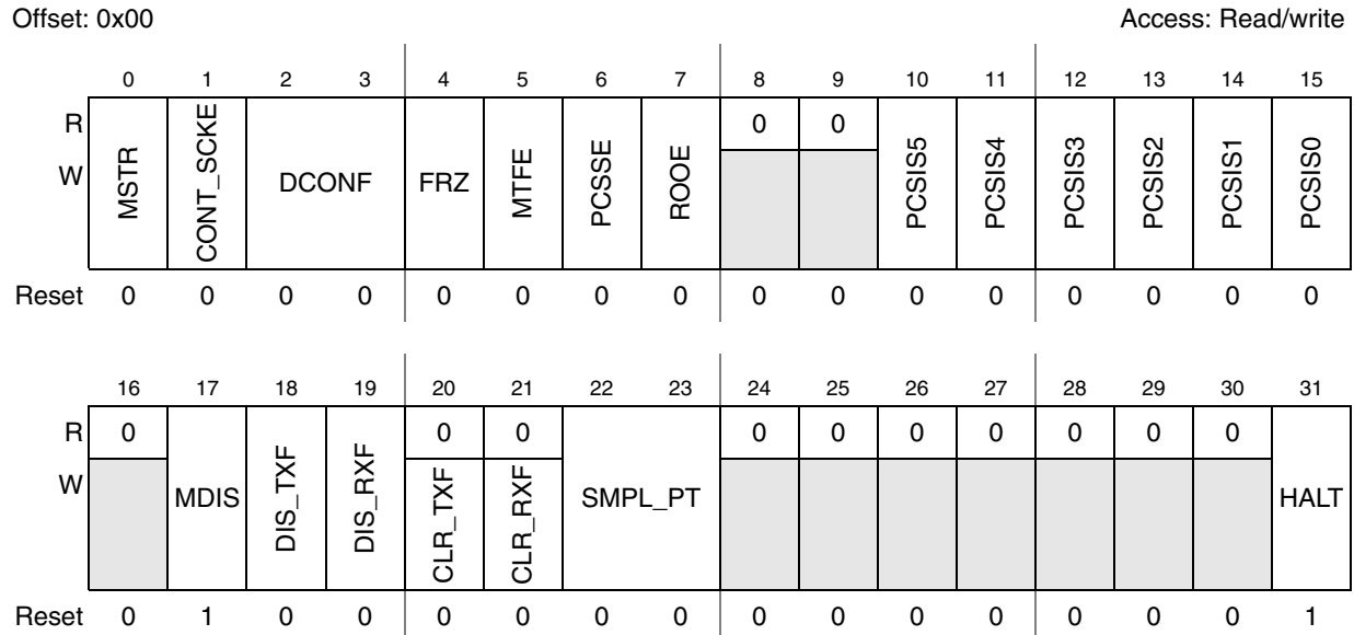
Figure 26-3. DSPI Module Configuration Register (DSPIx_MCR)
